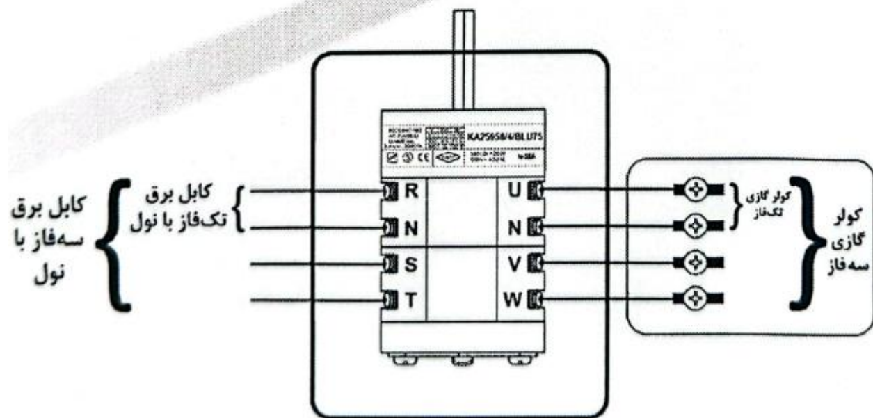
کلید ایزولاتور کولر گازی ۴ پل الکتروکاوچ (در کلیدهای ۲ پل، ترمینال های V, W / S, T وجود ندارد)
